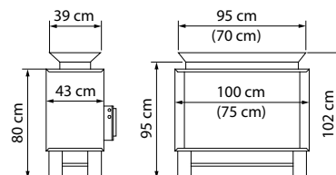
Volitelný upevňovací rám pro o 30 - 45 kg větší objem kamene. Volitelná vypínací kolébka s montáží přímo na kamna.
