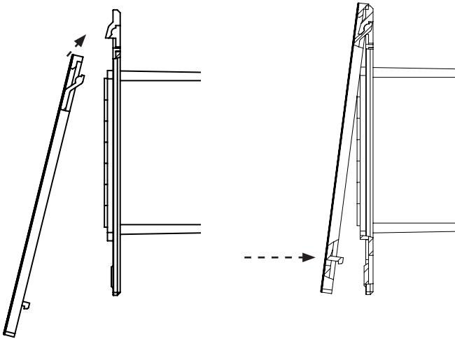
Obr. 7 Montáž ovladače
