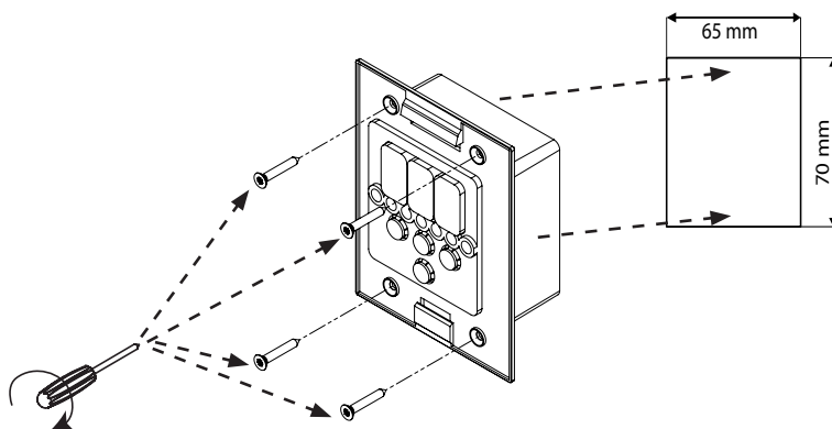
Obr. 5 Montáž ovladače Pro D
